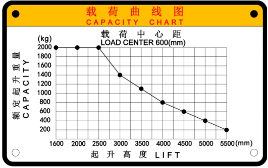
图 3-6-1 载荷曲线图 (三级门架)
