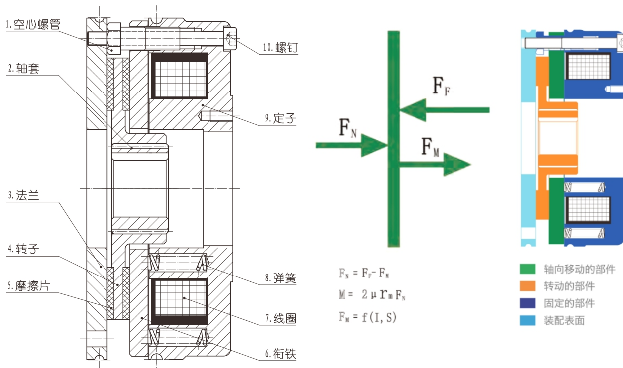
图 8-5 制动原理图
