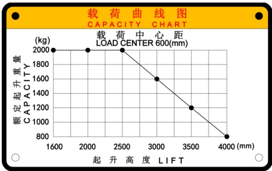
图 3-6-1 载荷曲线图
