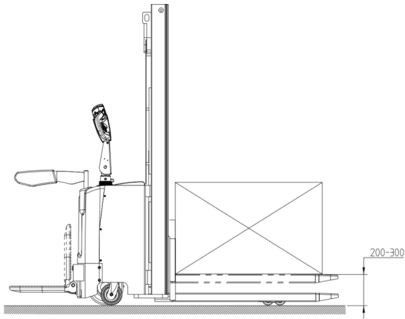
图 9 载荷示意图
