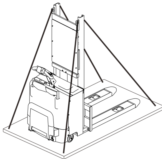
图 5-2-2 固定点
