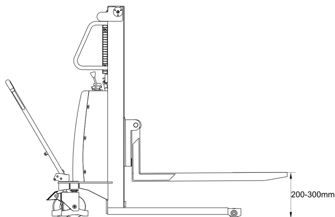
图 19 货叉离地 200mm-300mm
