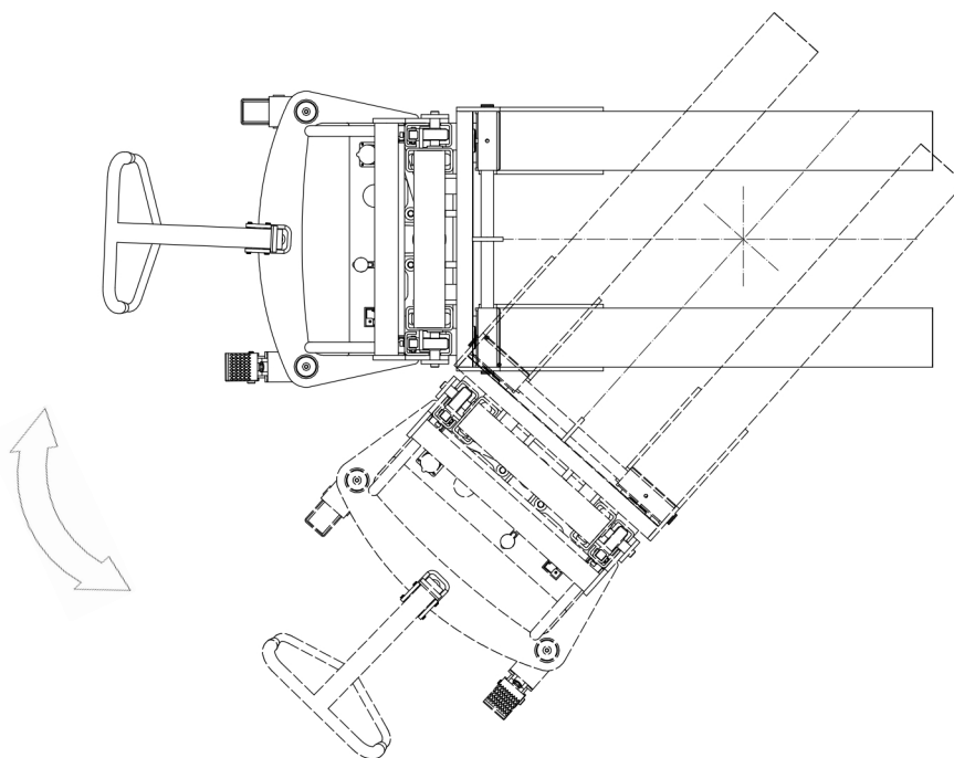
图 14 转弯轨迹示意图
