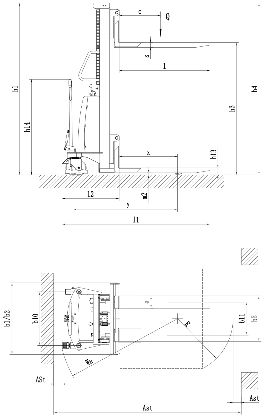
图 3 技术参数图
