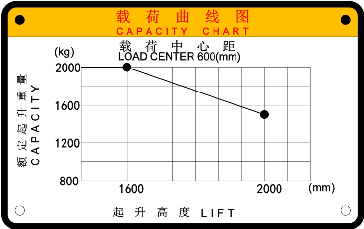
图 8 载荷曲线示意图 (2.0 吨)
