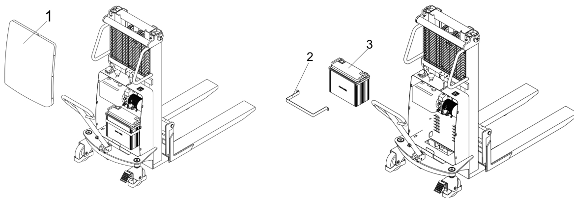
图 22 电池更换示意图
