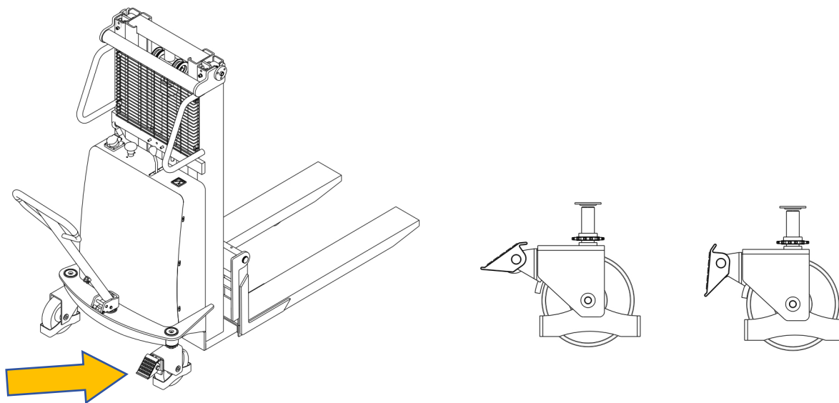
图 15 制动示意图
