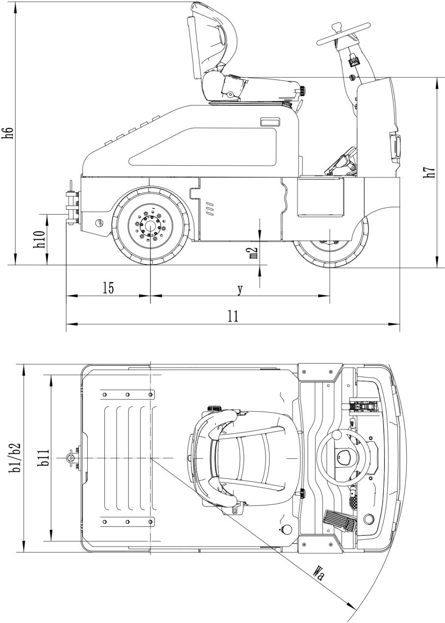
图 3 技术参数图
