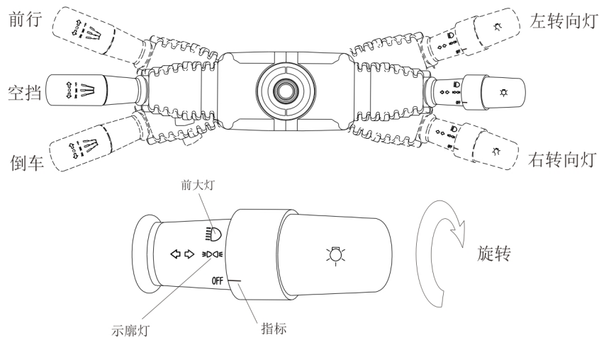
图 12 组合开关
