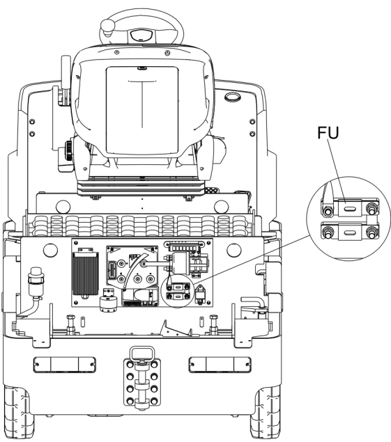
图 26 保险丝位置
