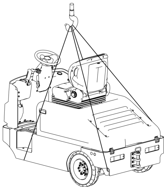
图 6 起吊
