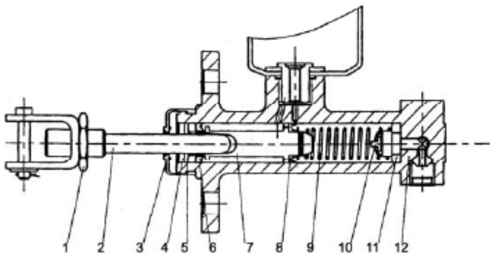
图 17 制动总泵示意图
