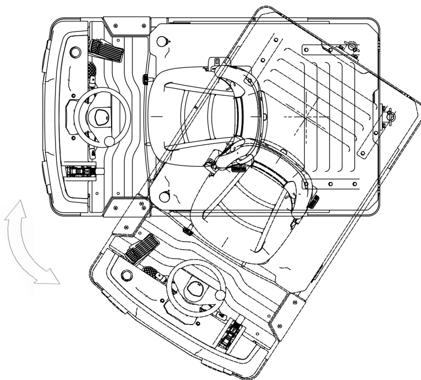
图 13 转向示意图
