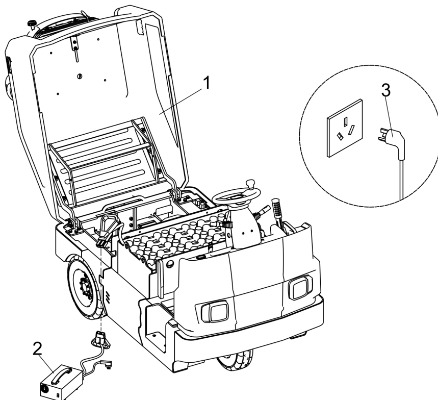
图 23 充电口位置示意图
