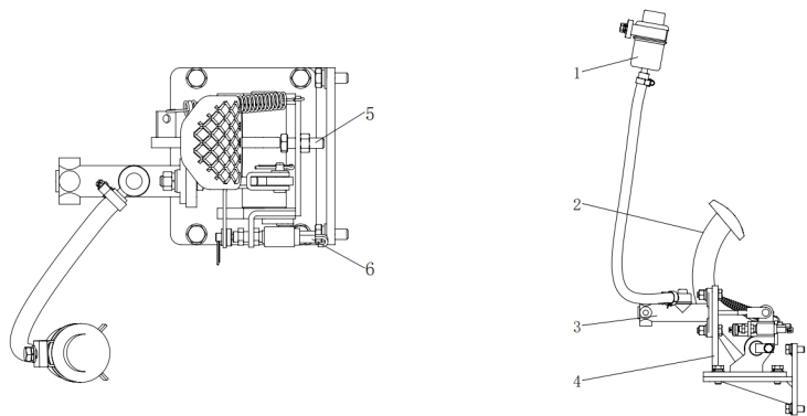
图 16 制动踏板示意图
