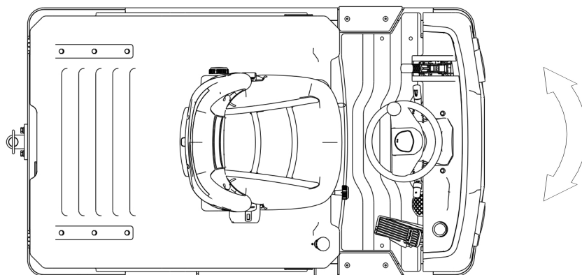
图 13 转向示意图
