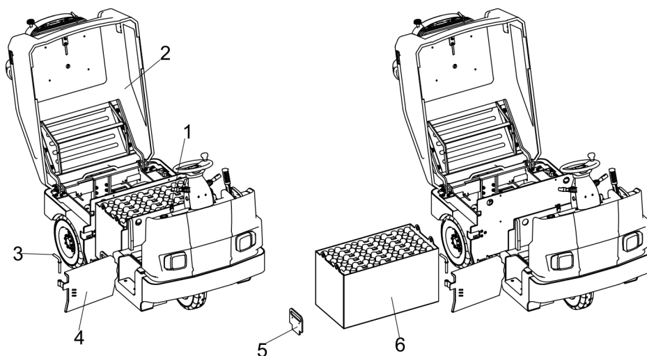
图 22 电池更换示意图
