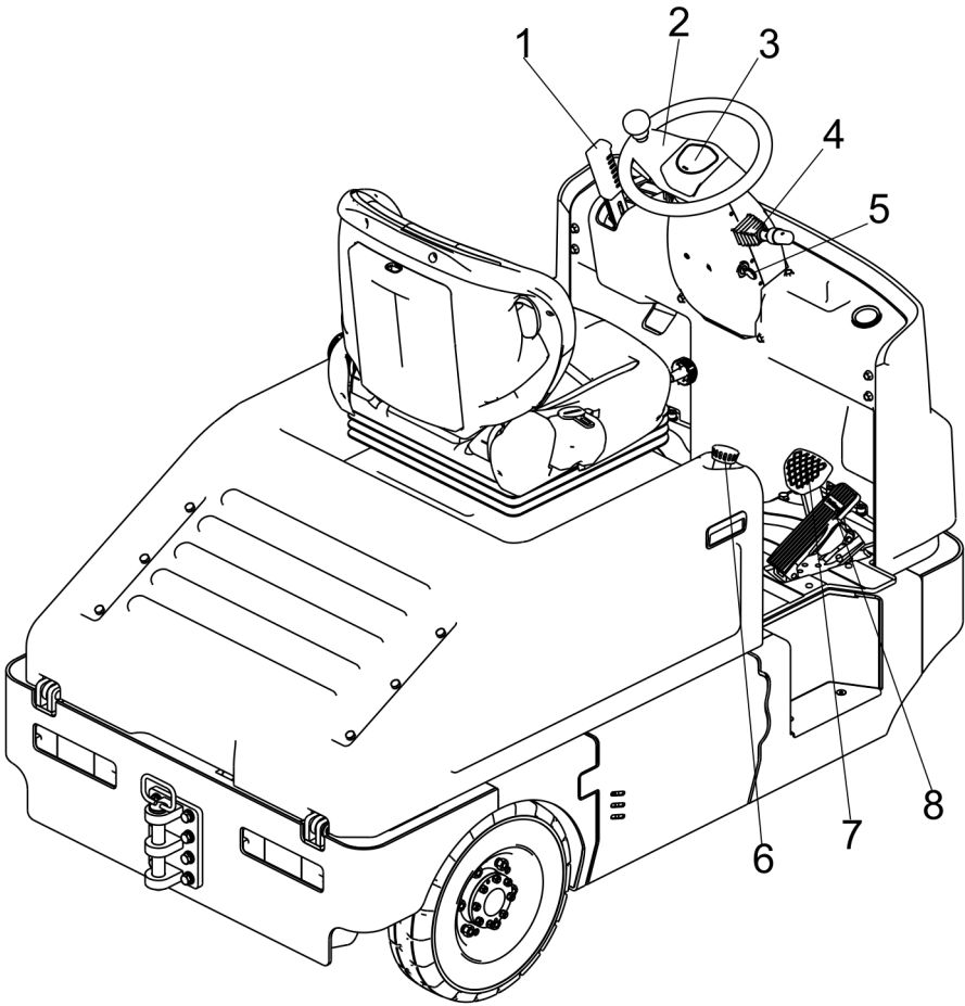
图 8 操作控制台
