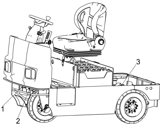
图 25 润滑点
